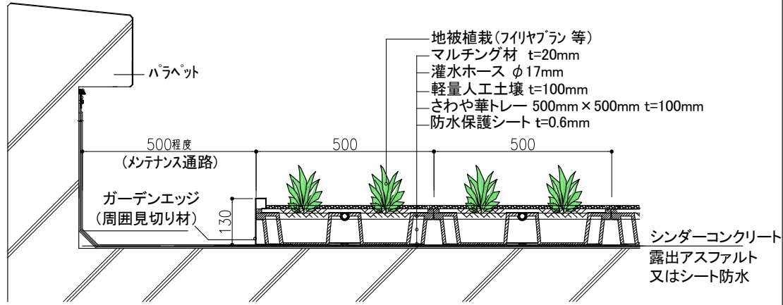
陸屋根標準納まり図
