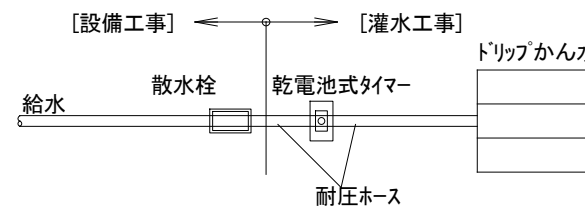
簡易型灌水システム系統図(乾電池式タイマー)
